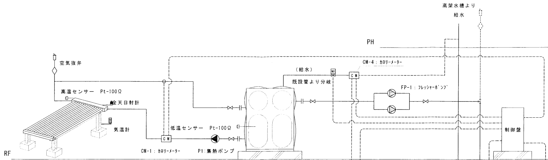
FSP: 太陽熱集熱器 41パネル
